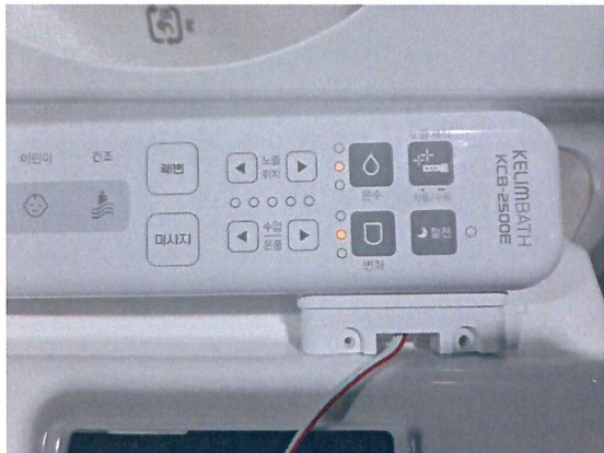
시험 전 제품 동작 확인 (3)
