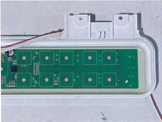
시험 후 제품 내부 사진 (7)
