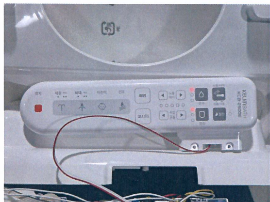
시험 후 제품 동작 확인 (4)
