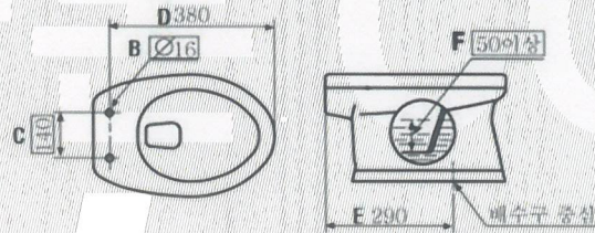
대변기 세척구
