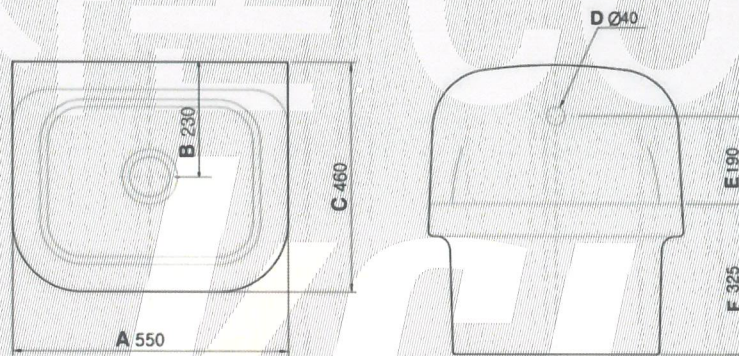
받이 달린 청소용 수채 S-125F(S210)
