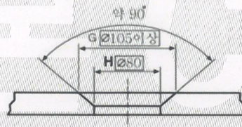
청소용 수채 배수구
