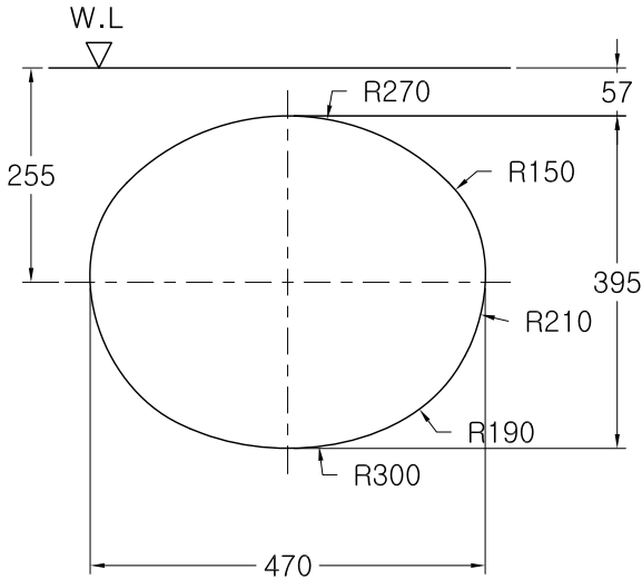
카운터절단규격
