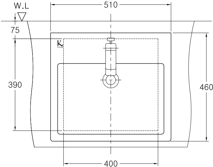
카운터 절단규격 (400X390)
