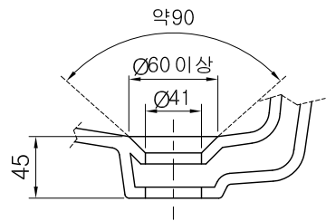
배수구 상세도 (2:1)
