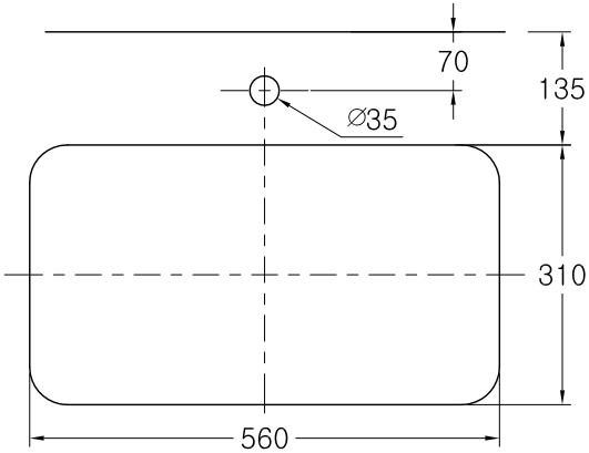
카운터절단 규격
