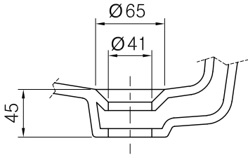
배수구 상세도 (2:1)
