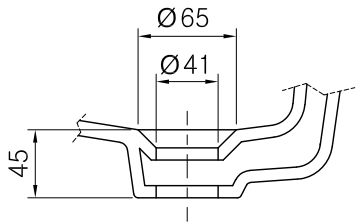
배수구 상세도 (2:1)
