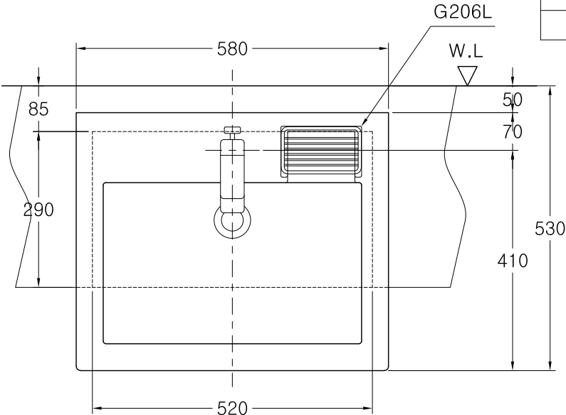
카운터절단규격 (520X290X55)
