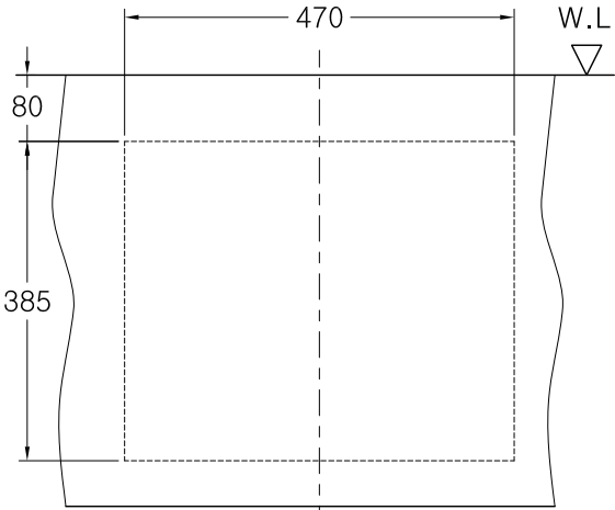
카운터절단규격
