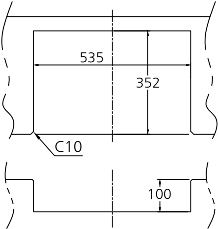
〈카운터 시공도〉
