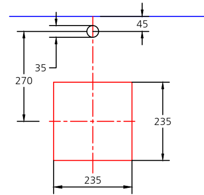
〈CL-822 타공도〉
