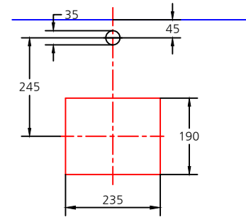
<CL-823 타공도>
