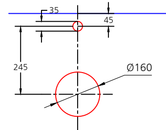
<CL-830 타공도>
