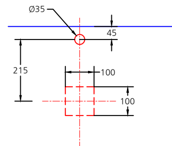
〈CL-840 타공도〉
