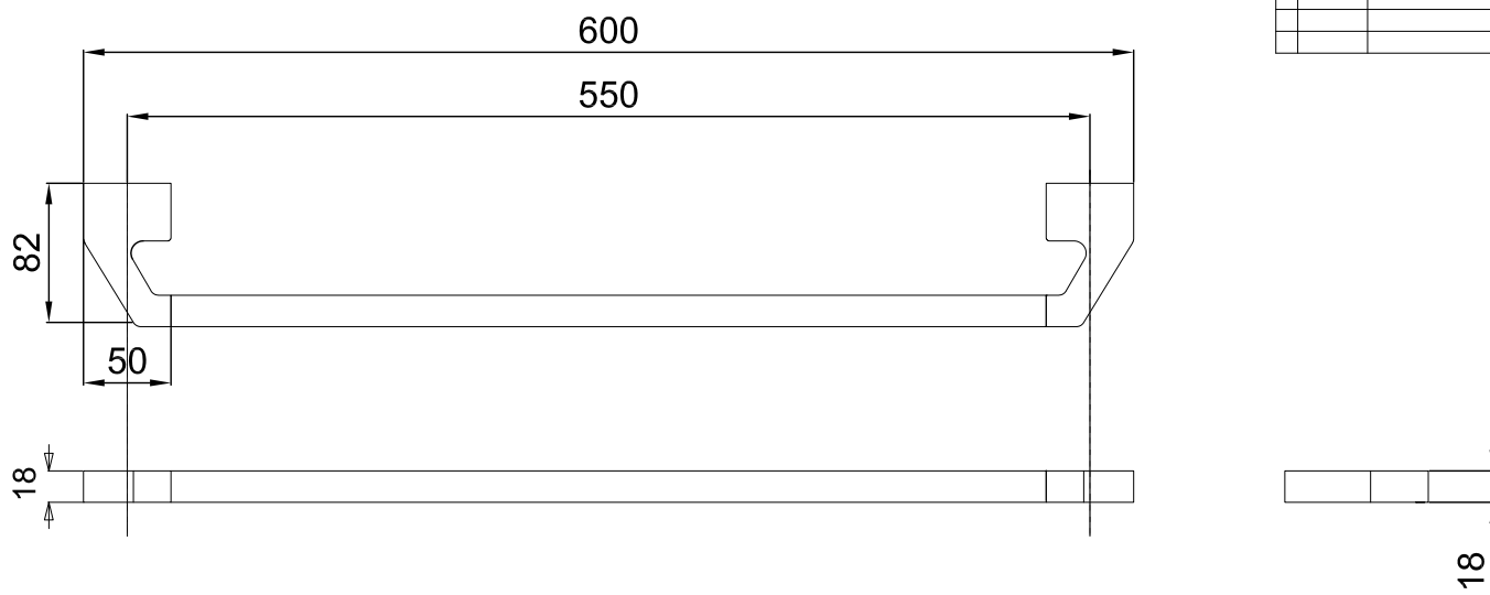
KCA-401
