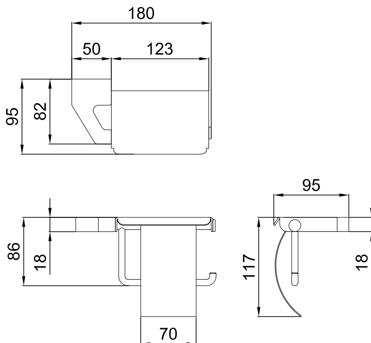
KCA-404
