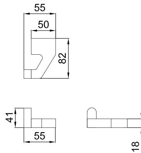
KCA-403
