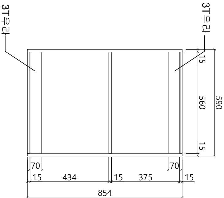
전 단 면 도
