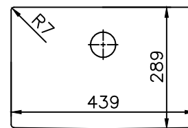
카운터 시공도
