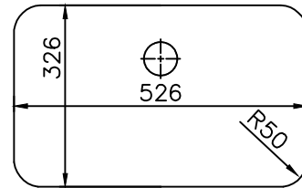
카운터 시공도
