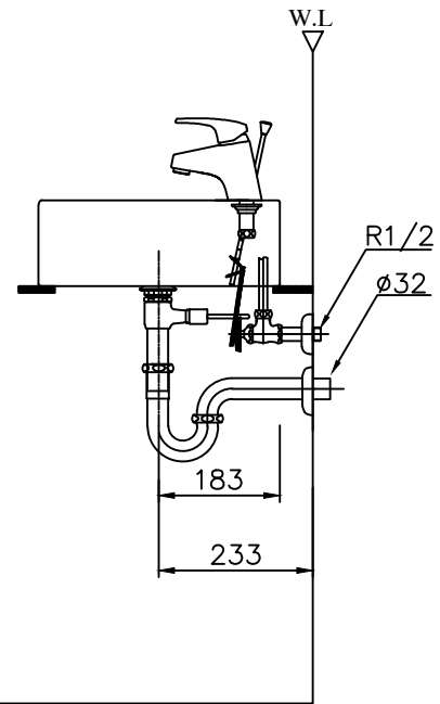
카운터 시공도
