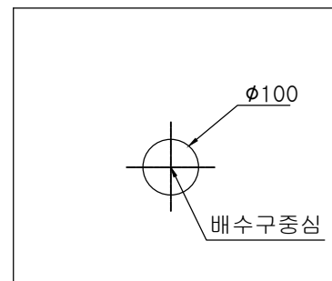
(설치구 가공도)
