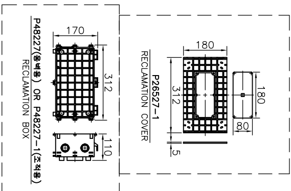
매립부 SCALE:1/8
