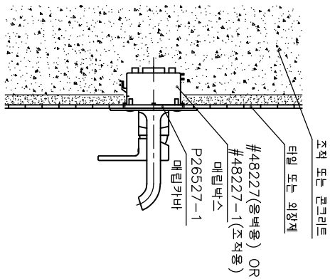
설치도 SCALE:1/8
