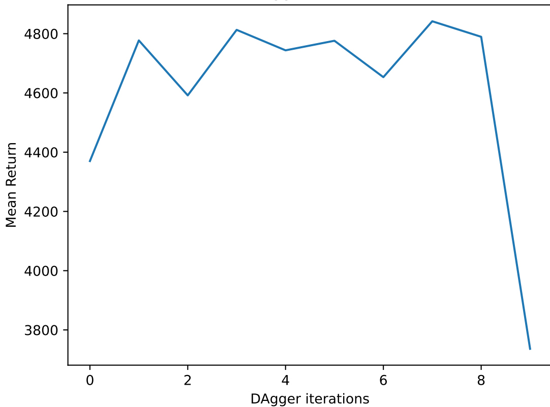
DAgger: Ant-v4
