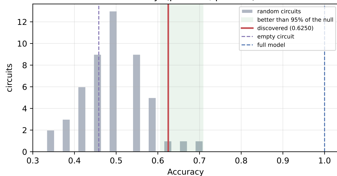
KL Div (pct 8.0, p 0.922)
