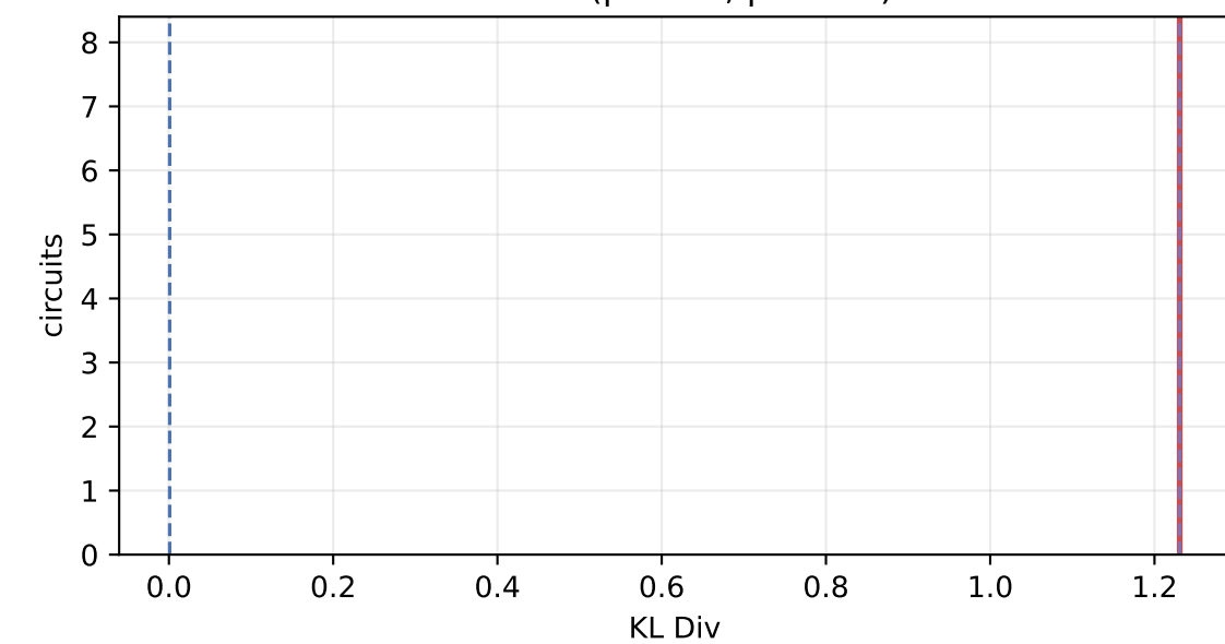
KL Div (pct 2.0, p 0.980)
