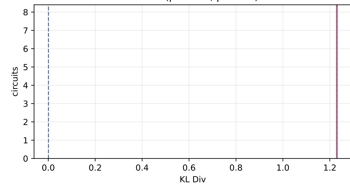
KL Div (pct 48.0, p 0.529)
