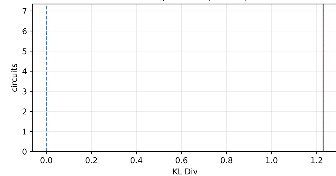
KL Div (pct 20.0, p 0.804)
