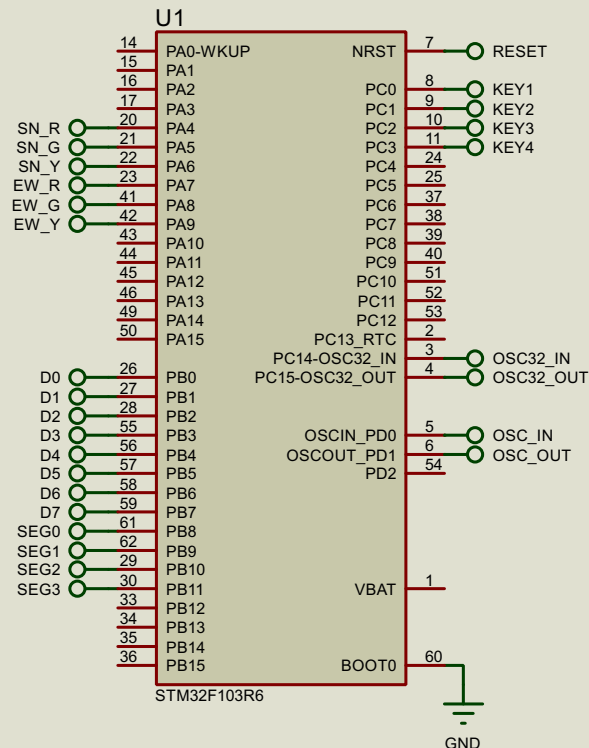
交通灯主控电路
