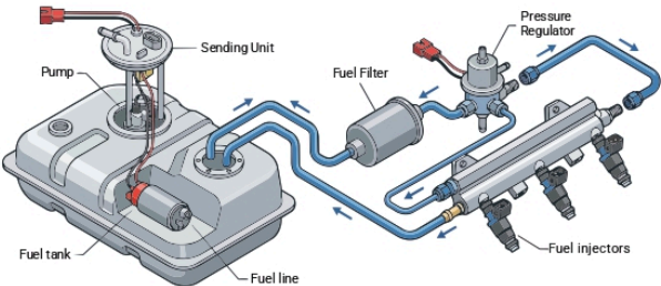
FUEL SYSTEM 燃油系统
