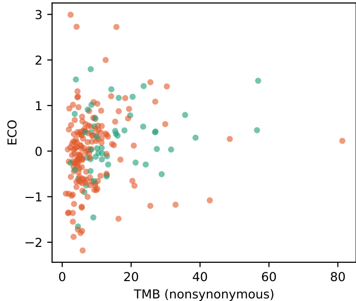
A. ECO vs TMB ( \rho=0.26 , p=0.000 )
