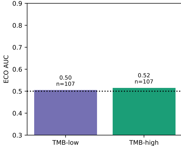
B. ECO within TMB strata
