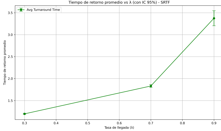
Figura 3: Tiempo de retorno promedio vs tasa de llegada \lambda con IC 95 %
