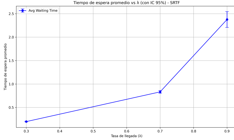
Figura 2: Tiempo de espera promedio vs tasa de llegada ( \lambda ) con intervalo de confianza del 95 %).
