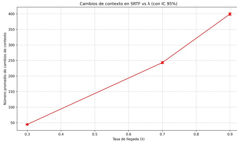
Figura 5: Número promedio de cambios de contexto vs tasa de llegada ( \lambda ) con intervalo de confianza del 95 %.
