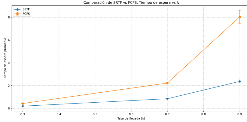
Figura 6: Comparación de tiempo de espera entre SRTF y FCFS
