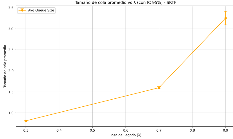
Figura 4: Tamaño de cola promedio vs tasa de llegada \lambda con IC 95 %
