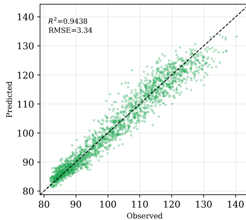
GRU
