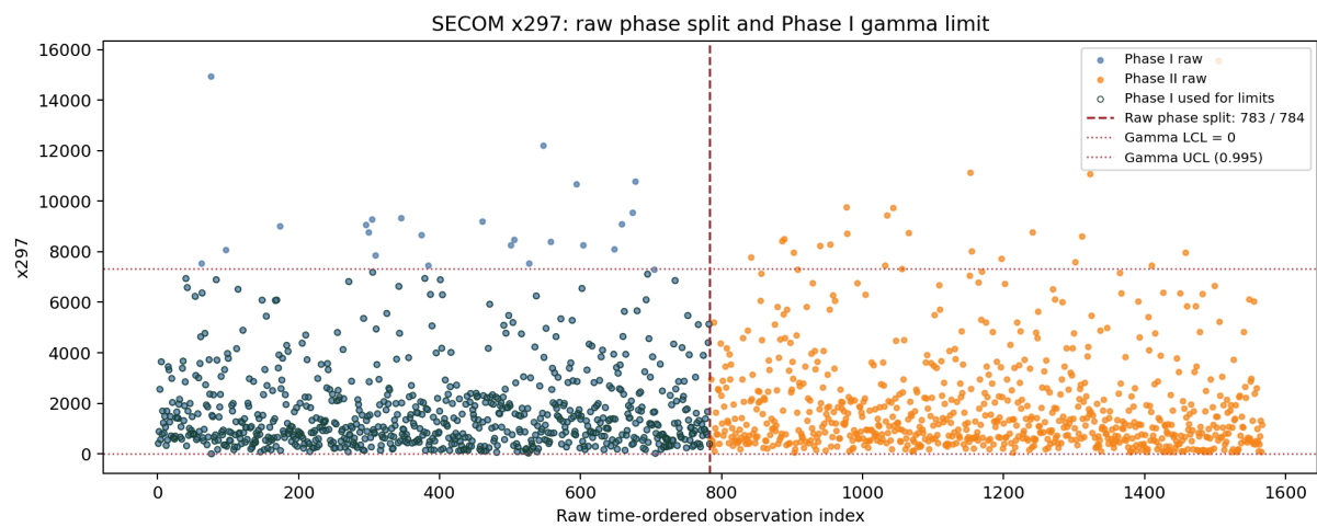
圖 2.1: 原始資料切分與 Phase I Gamma 管制界線
