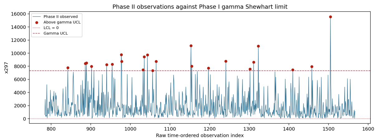
圖 3.1: Phase II 觀測值與 Gamma Shewhart 上管制界線
