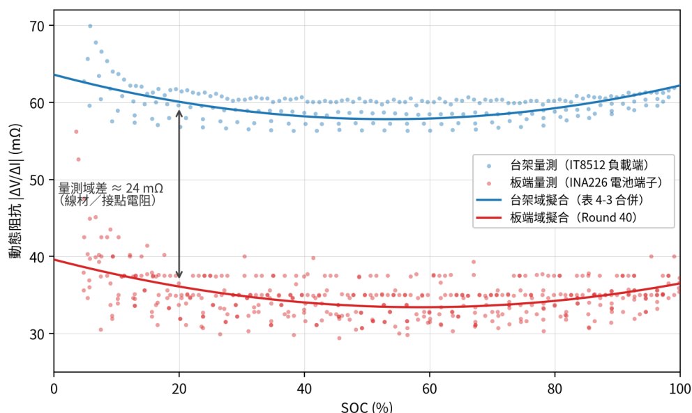
圖 4-5 動態阻抗之量測域對照：台架（IT8512 負載端）與板端（INA226 電池端子）之 |\Delta V/\Delta I| -SOC 散點及各自域內二次擬合（兩域斜率項幾乎相同、常數項相差約 24 mΩ 之線材／接點電阻）
