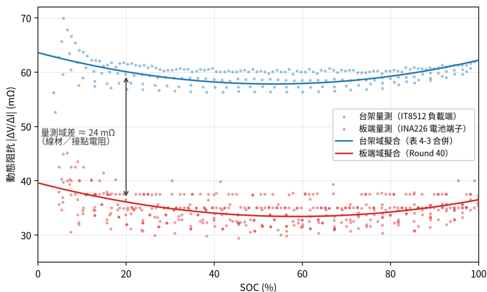
圖 4-5 動態阻抗之量測域對照：台架（IT8512 負載端）與板端（INA226 電池端子）之 |ΔV/ΔI| -SOC 散點及各自域內二次擬合（兩域斜率項幾乎相同、常數項相差約 24 m \Omega 之線材／接點電阻）
