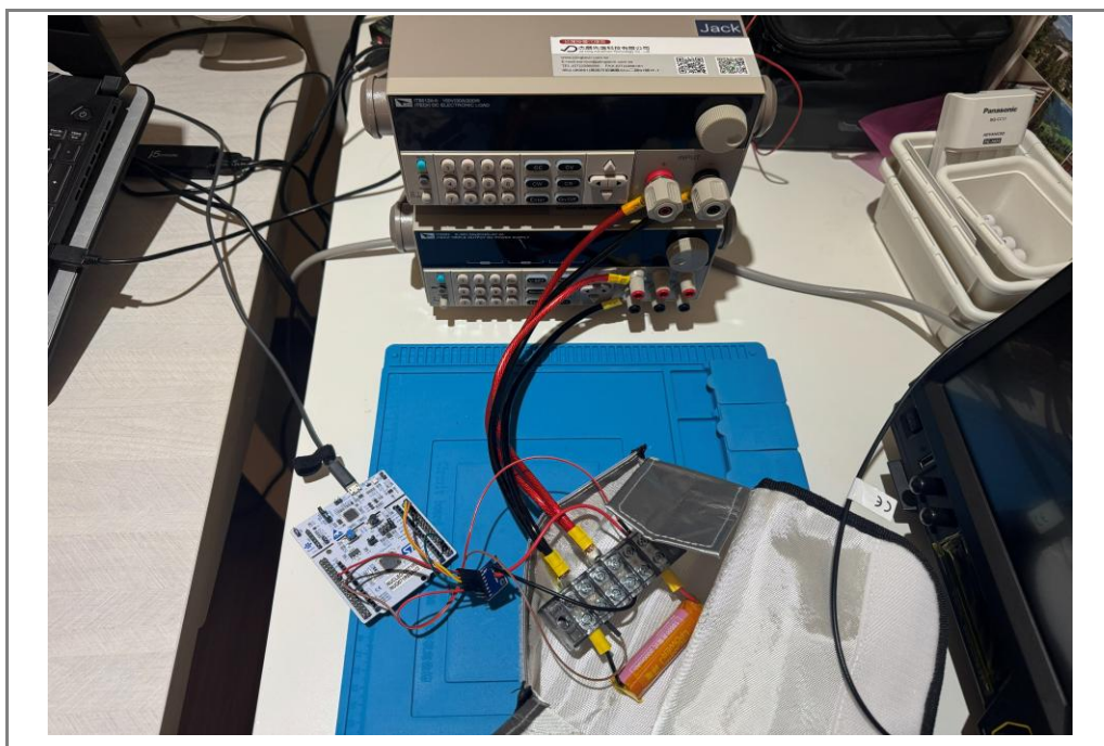
圖 3-3 測試平台實際外觀：可程式電源、電子負載、受測電池與嵌入式量測板之實體配置
