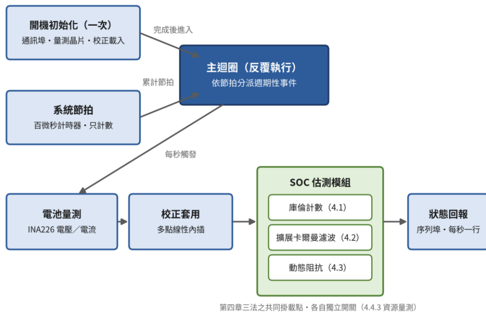
圖 3-4 韌體骨架與三種 SOC 估測方法之掛載關係
