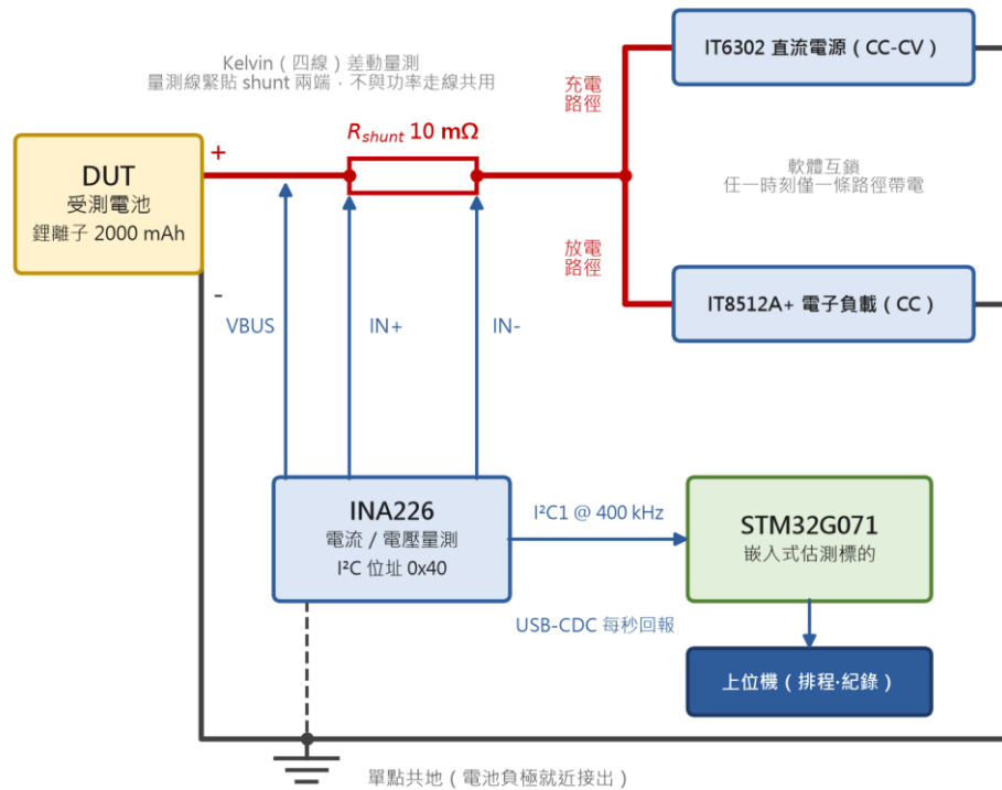
圖 3-2 量測迴路接線圖：電池正極經 10\text{ m}\Omega shunt 分接至電源與電子負載兩條互斥路徑，INA226 以 IN+/IN- 跨接 shunt 兩端量測電流、VBUS 量測電池端點電壓，並自電池負極單點共地
