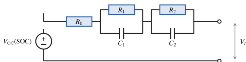
(c) 二階 RC 模型
