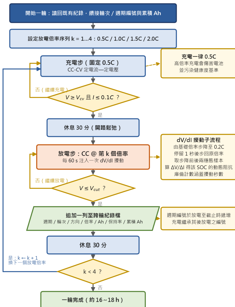
圖 3-5 跨輪自動化測試協定流程：一輪依序執行四組「充電 → 休息 → 放電 → 休息」，充電固定 0.5C 並以 CC-CV 終止條件判斷充飽，放電每 60 s 注入一次 dV/dI 擾動，每步結束即追加一列跨輪紀錄，四種放電倍率跑完為一輪
