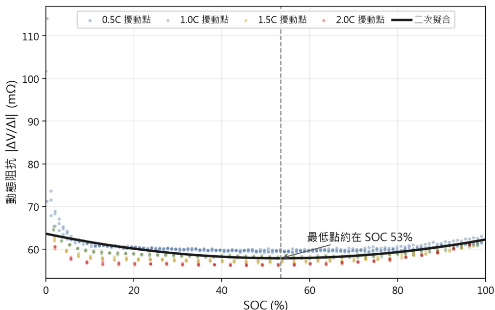
圖 4-4 動態阻抗 |\Delta V/\Delta I| 隨 SOC 之實測散點與二次擬合（fresh-cell rounds 1–3，四種放電倍率）
