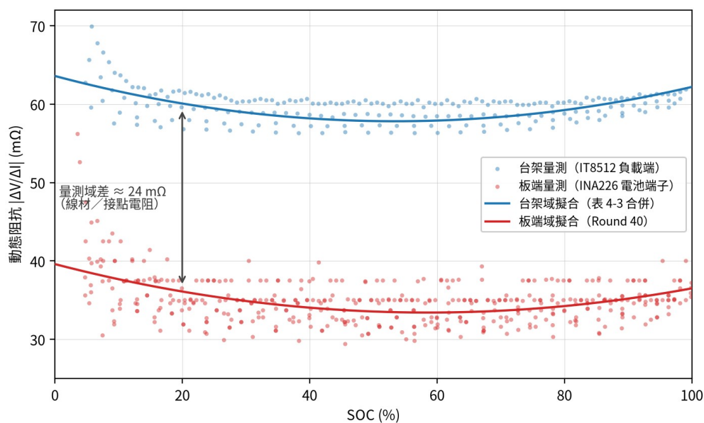
圖 4-5 動態阻抗之量測域對照：台架（IT8512 負載端）與板端（INA226 電池端子）之 |\Delta V/\Delta I| -SOC 散點及各自域內二次擬合（Round 40；兩域斜率項幾乎相同、常數項相差約 24 mΩ 之線材／接點電阻）
