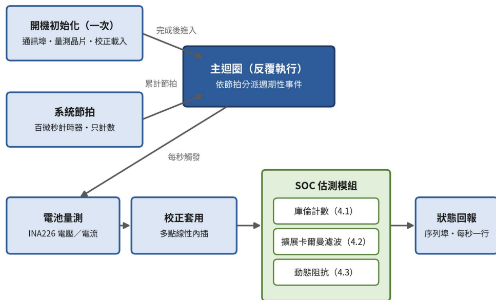
第四章三法之共同掛載點・各自獨立開關（4.4.3 資源量測）
