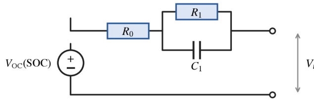
(b) 戴維寧（一階 RC）模型
