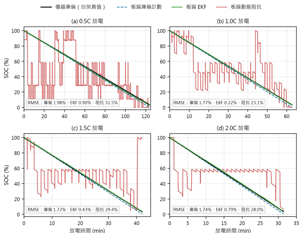
圖 4-6 三法 SOC 估測軌跡與台架庫倫真值之對照 (Round 41 板端實測，四種放電倍率；各面板標註對台架真值之 RMSE)
