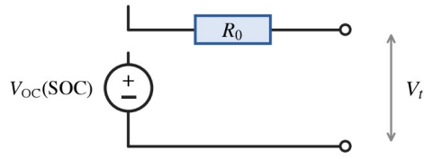
(a) 內阻模型
