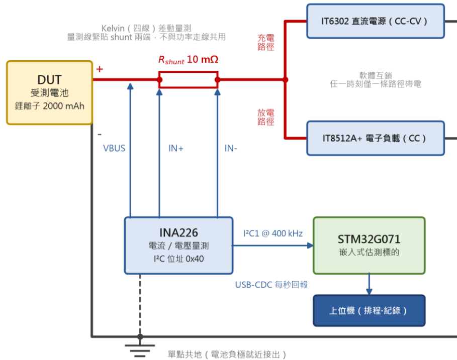
圖 3-2 量測迴路接線圖：電池正極經 10 mΩ shunt 分接至電源與電子負載兩條互斥路徑，INA226 以 IN+／IN- 跨接 shunt 兩端量測電流、VBUS 量測電池端點電壓，並自電池負極單點共地
