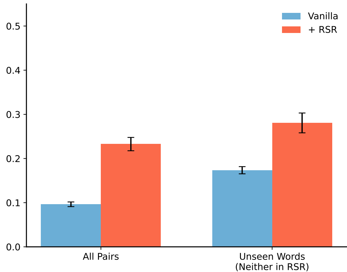
GPT-2
