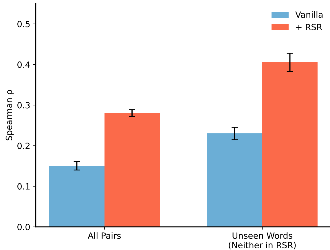
BERT
