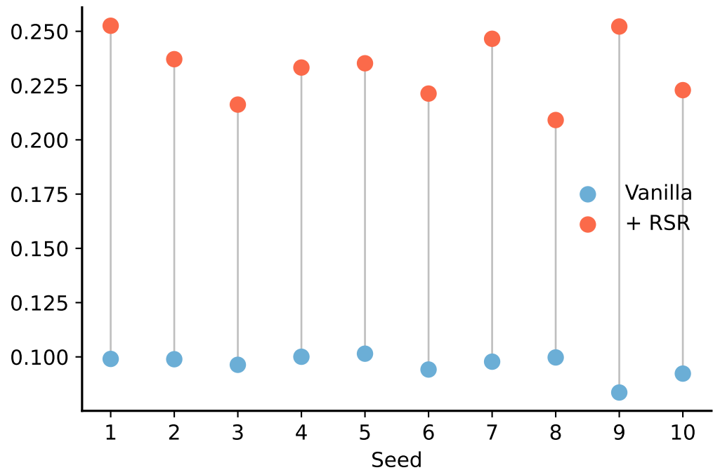
GPT-2
