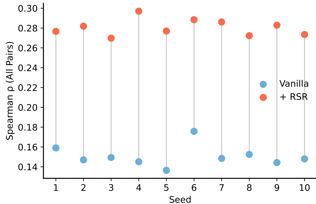
BERT
