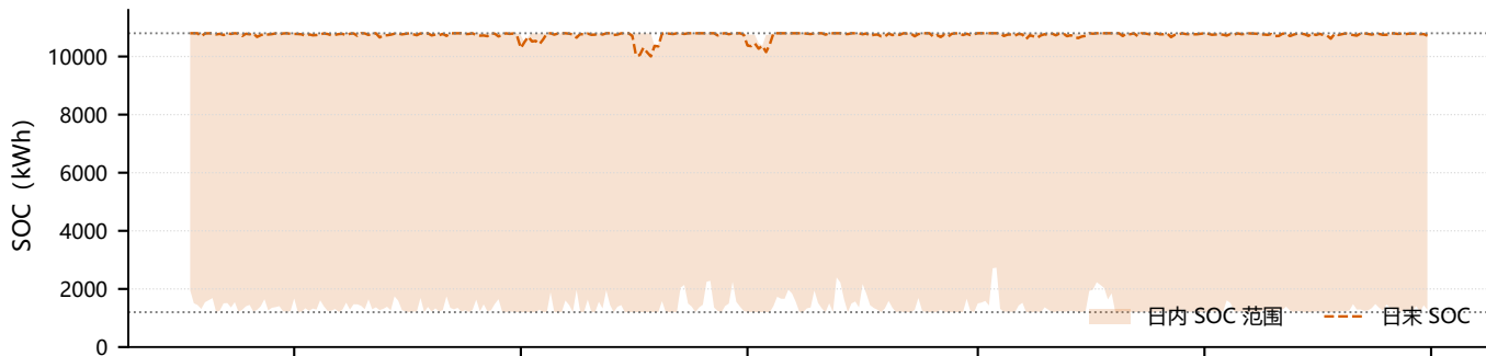
两种执行策略的跨日 SOC 连续轨迹
