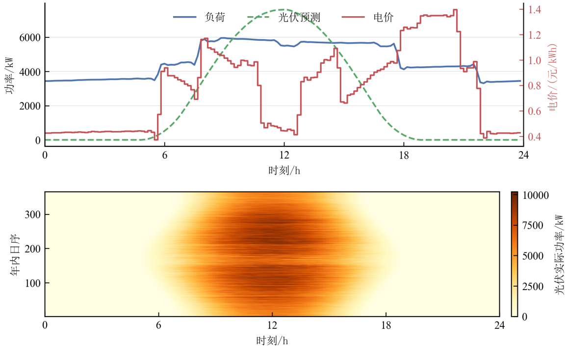
图 2: 微网典型日与全年负荷、光伏数据全景
