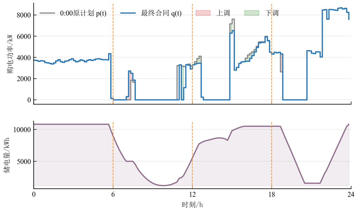
图 10: 问题三代表日的事件驱动合同调整与 SOC 轨迹
