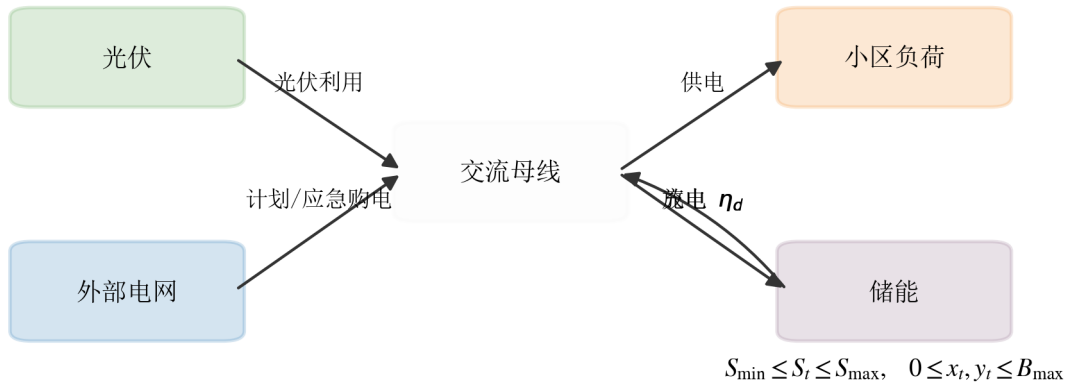
图 3: 微网能量流与储能约束示意图
