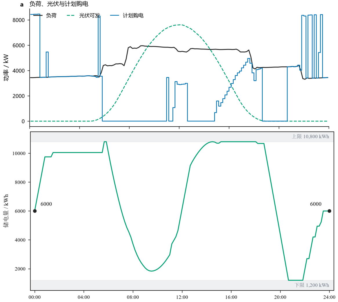
图 4: 问题一最优购电调度与储能状态轨迹
