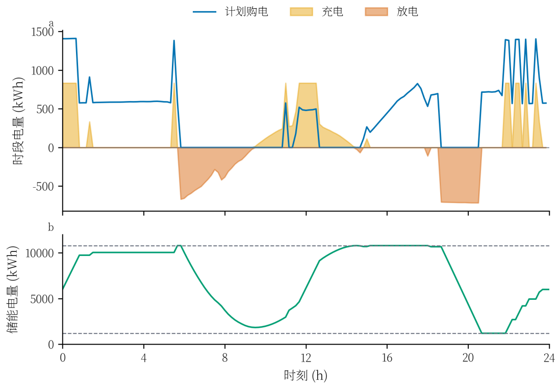
图 1: 典型日购电、充放电与储能状态
