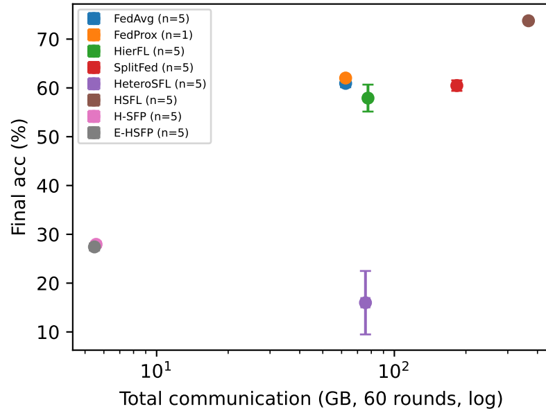
cifar10
