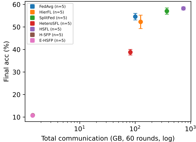
cifar100
