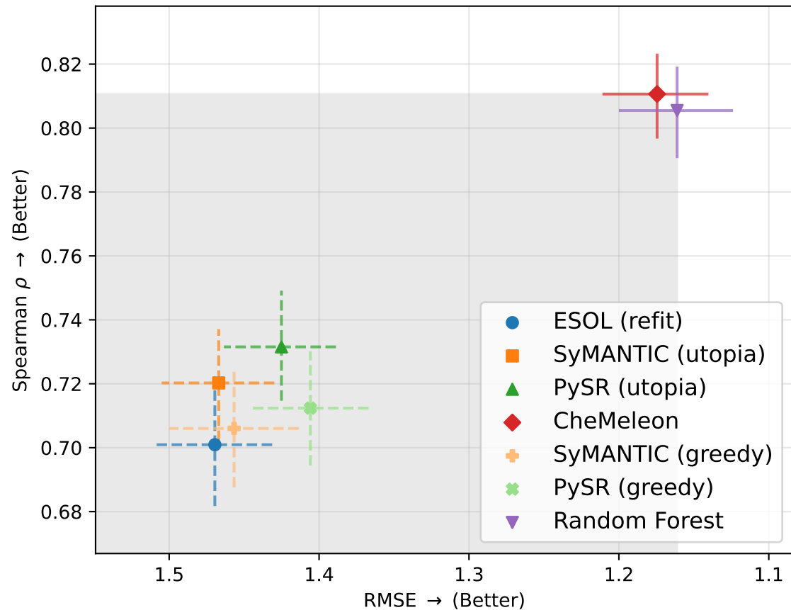
OChem
