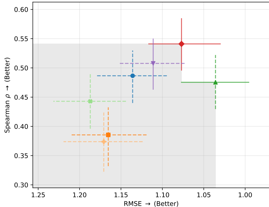
Biogen
