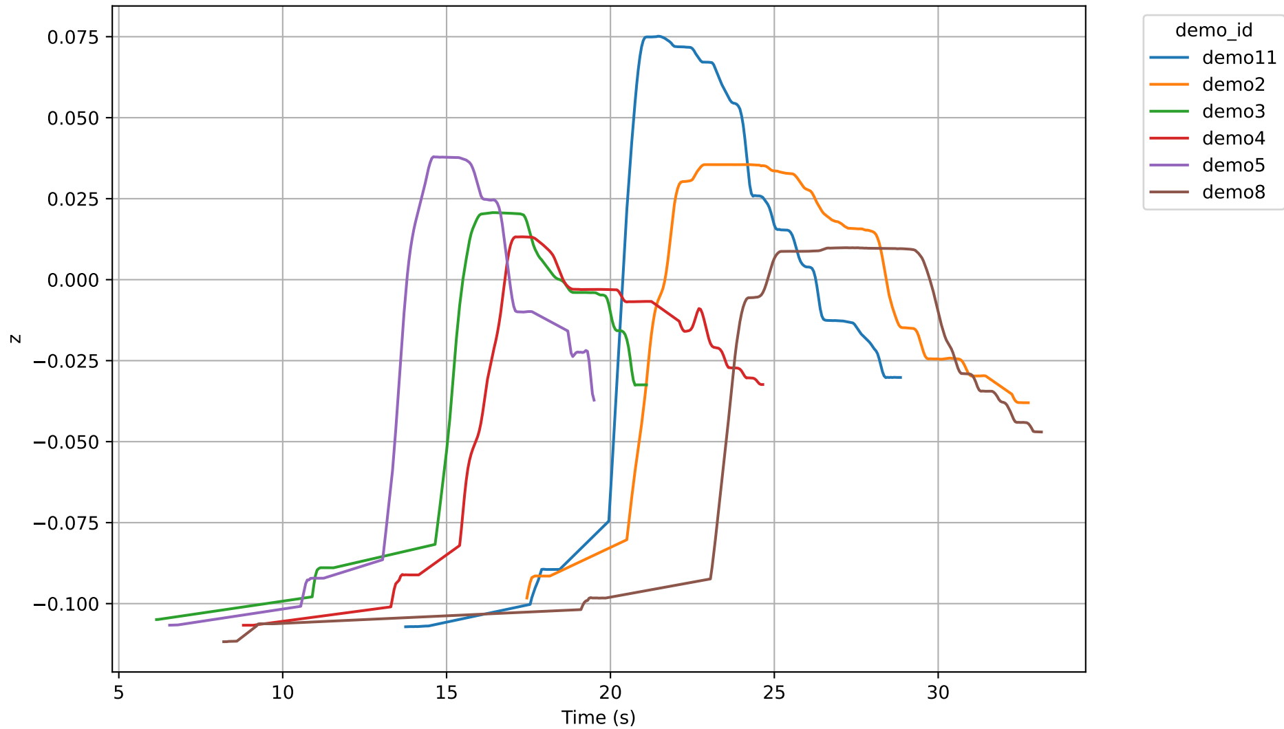
Min1 → Min2 Z Trajectories Over Time
