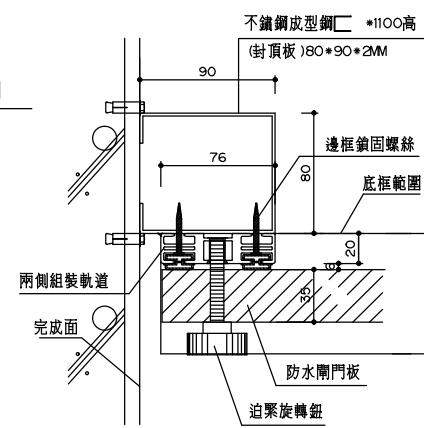
邊框大樣之C詳圖
