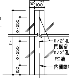
RC 邊框大樣 牆面嵌板安裝立面圖
