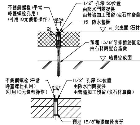
詳圖H(地面固定法大樣) RC 地坪面鑽孔安裝示意圖 N.T.S. UNIT:mm 4
