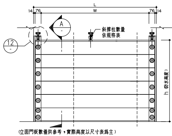
防水閘門立面示意圖--單片式
