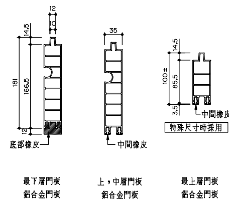
門板詳圖 N.T.S. UNIT=mm 5
