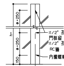
RC 邊框大樣之詳圖 A 牆面嵌板安裝立面圖
