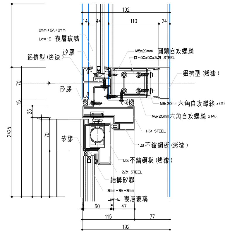
帷幕牆斷面詳圖
