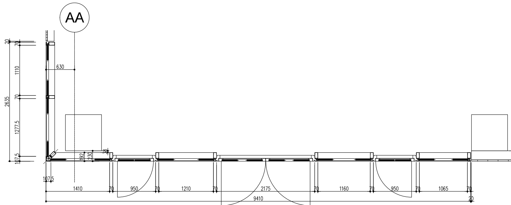
帷幕牆平面詳圖
