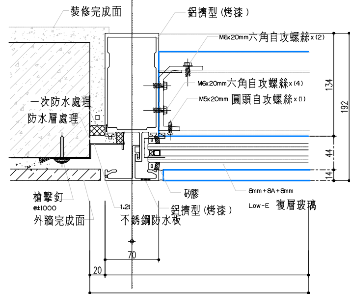
帷幕牆斷面詳圖
