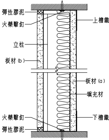
TYPE C 纖維水泥板 (雙面)管道間 N.T.S. UNIT:mm 5
