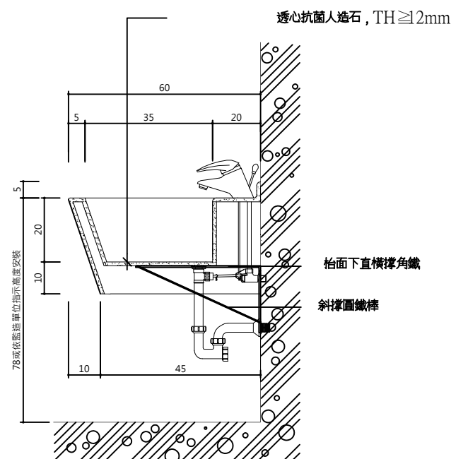
浴廁洗手枱剖面圖
