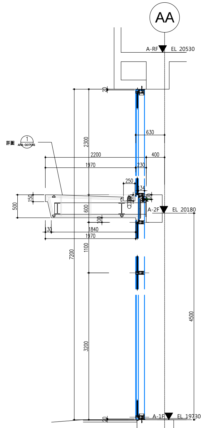
帷幕牆及入口雨遮剖面圖
