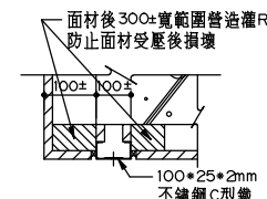
邊框大樣 未使用中示意圖
