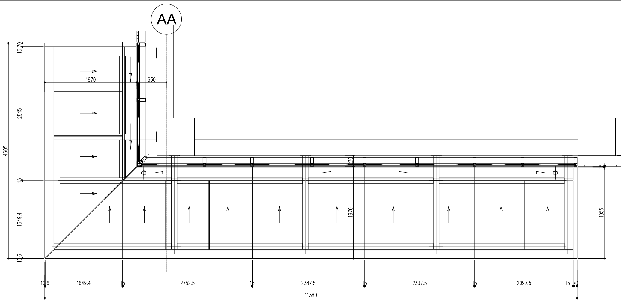
入口雨遮平面詳圖
