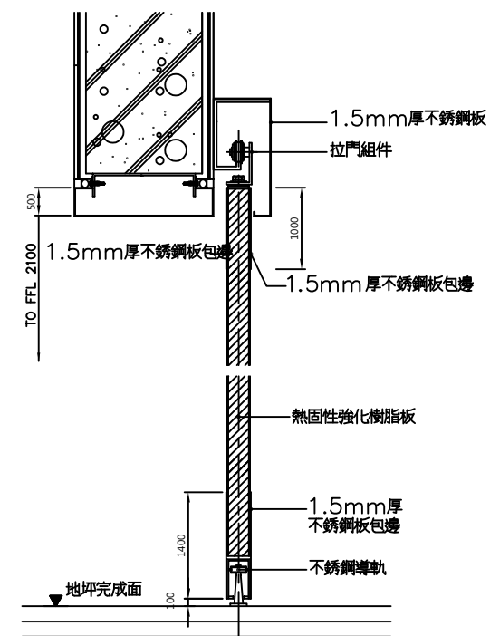
橫拉門詳圖
