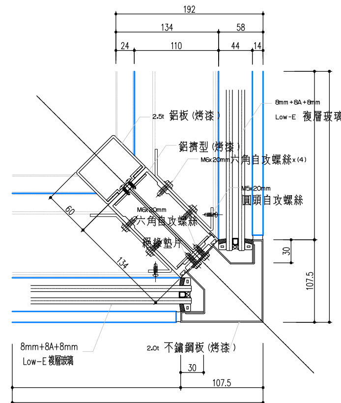
帷幕牆斷面詳圖
