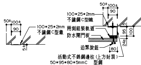
邊框大樣 未使用中示意圖
