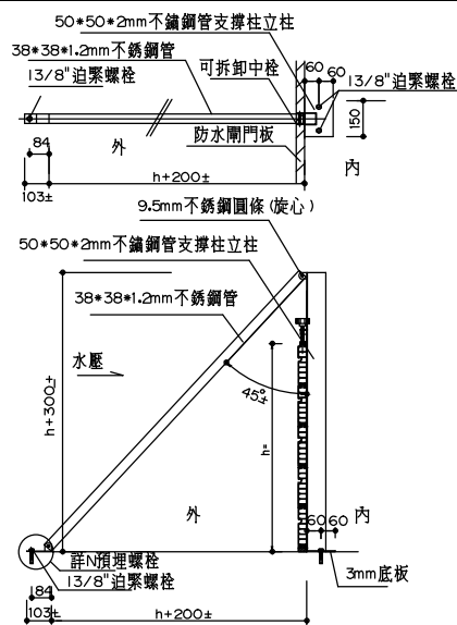
詳圖支撐柱(外拉式) 裝大樣--使用中
