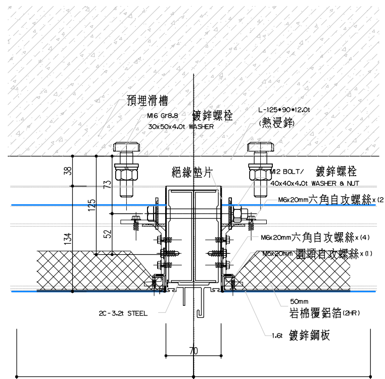
帷幕牆斷面詳圖
