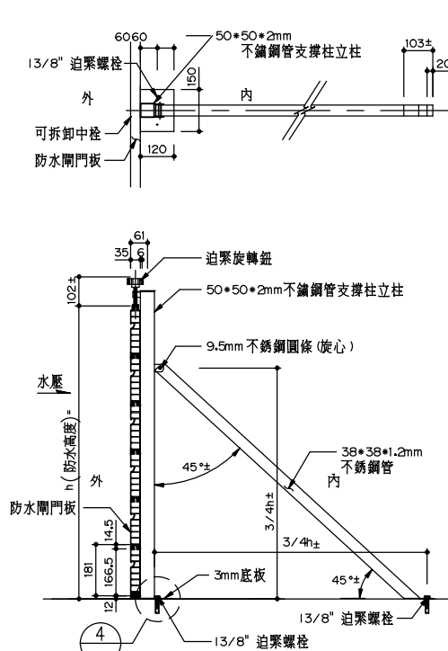
防水閘門立面示意圖--多片式
