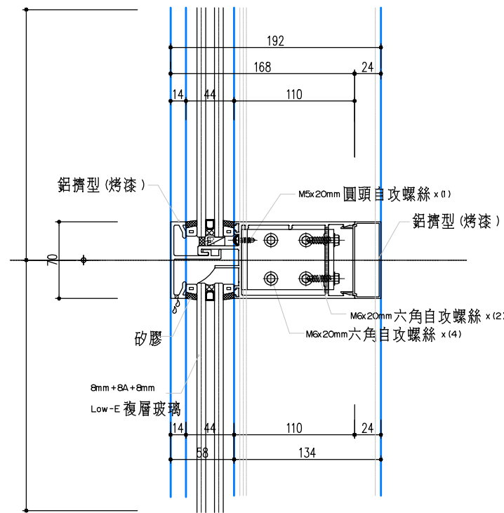
帷幕牆斷面詳圖
