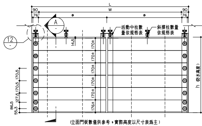
防水閘門立面示意圖--多片式
