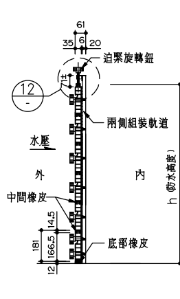
A-A剖面示意圖 N.T.S. UNIT:mm 3
