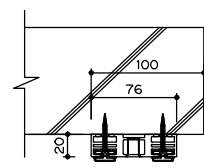
邊框大樣之C詳圖
