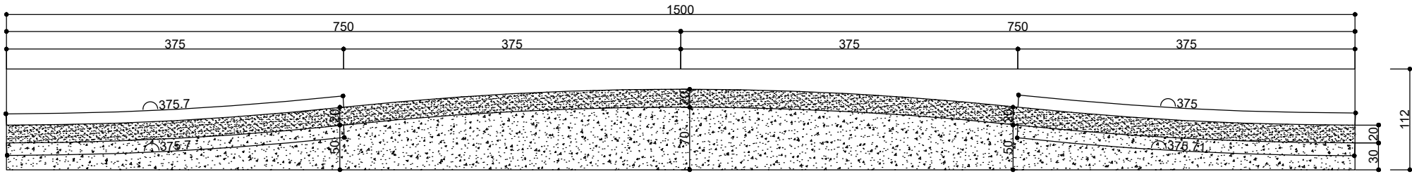
碼頭區RC護欄圖騰單元立面圖 1:60 UNIT=mm
