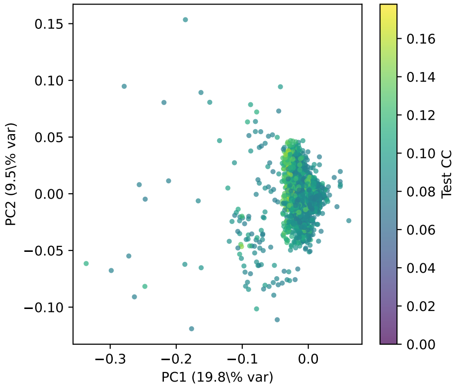
s3: Top-5\% Voxels — Functional PCA
