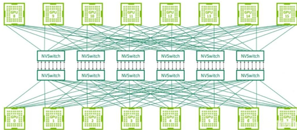
图表：NVLink交换系统
