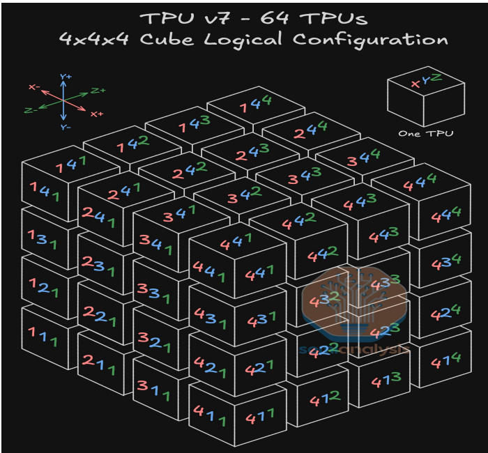
图表：谷歌TPU v7集群基础单元及芯片互连方式
