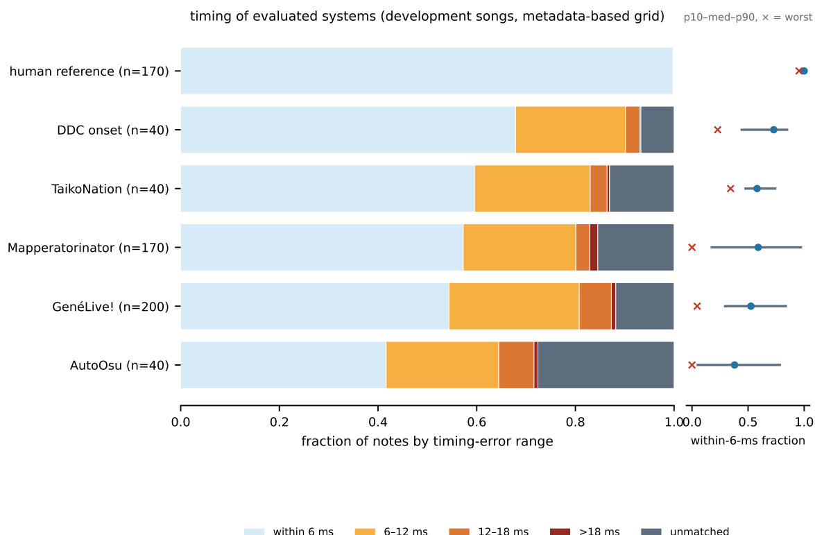
圖 5: 受評系統在 40 首發展歌曲上的時值，使用作者編定格線。每條顯示落在 6 ms 內、6–12、12–18、18 ms 以上或未配對的平均音符比例； n 為譜數。右側顯示 6 ms 內比例的第 10 百分位、中位數、第 90 百分位與最差譜面。
