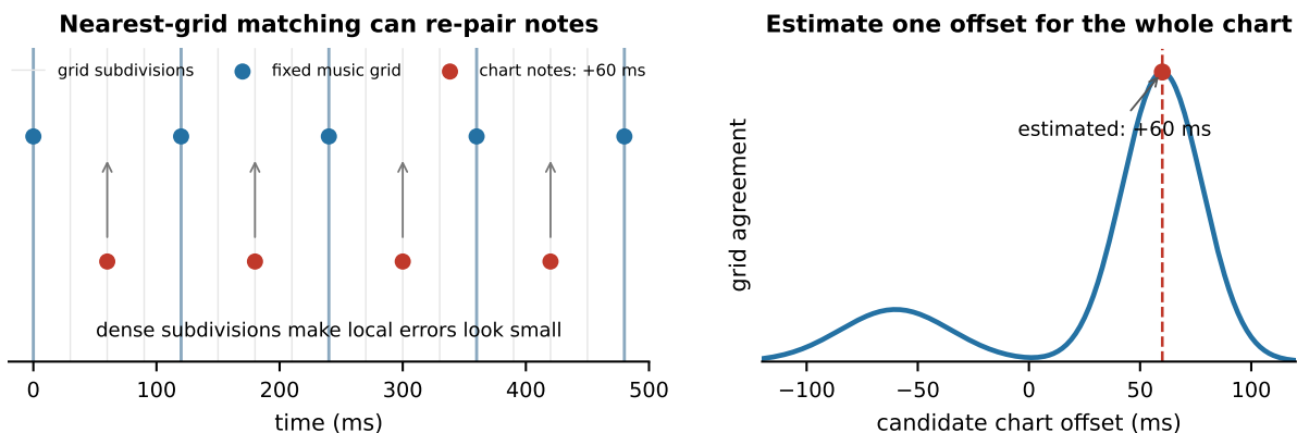
圖 2: 為何時值需要整譜估計。左: 最近格點配對可能把被平移的音符配到不同細分點、報出很小的局部誤差。右: 我們測試候選的整譜偏移, 選擇格線一致性最強者。格線如圖 1。
