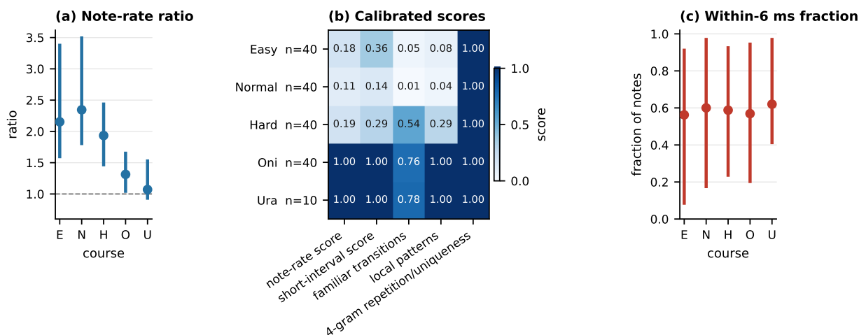
圖 6: Mapperatorinator 在配對發展譜上的探索性難度 profile。Easy 至 Oni 各含 40 個歌曲–course 配對；Ura 含 10 個。(a) 與 (c) 的點為中位數，豎線跨第 10 至 90 百分位。(a) 生成 / 人類音符率比；1 表示密度相等。(b) 依宣告角色分列的 calibrated score 中位數：四欄 band-typicality，1 表示位於範圍內，另一欄單側轉移熟悉度、越大越好。(c) 音符落在作者編定格線 6 ms 內的比列。
