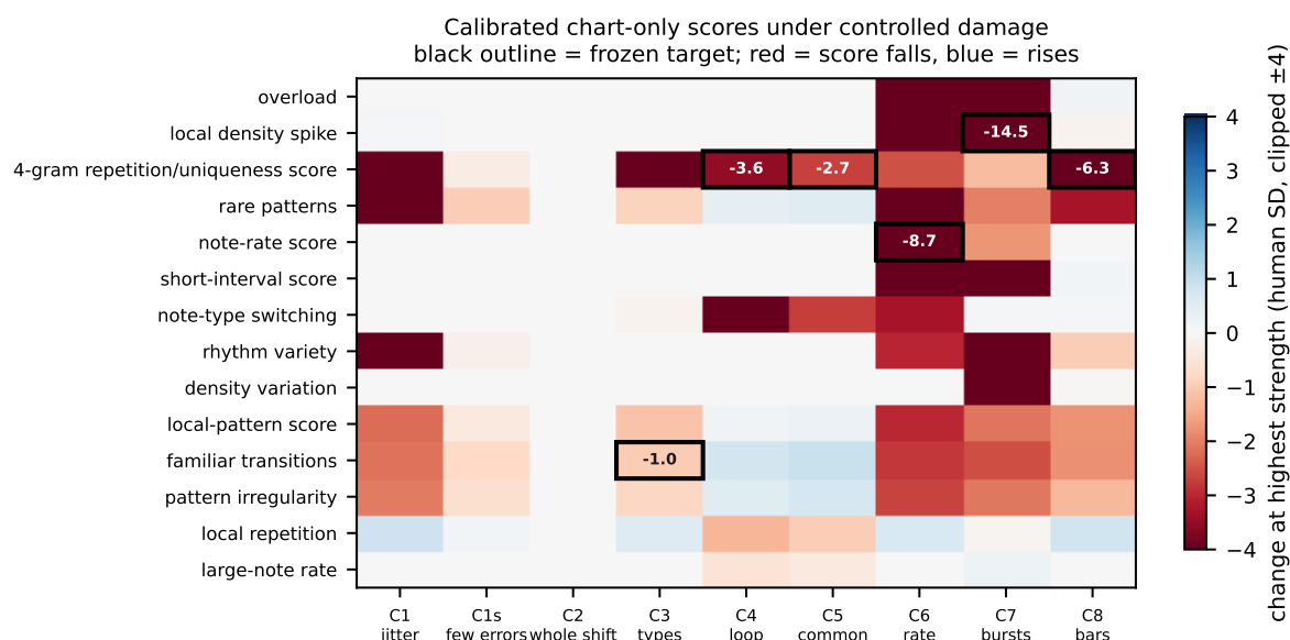
圖 4: 14 個非冗餘 calibrated chart-only scores 對各損壞在發展組最大強度下的反應，涵蓋 band-typicality scores 與單側 checks。紅色表示分數下降、藍色表示上升；數值以人類參照譜的標準差為單位，截斷於 \pm 4 。黑框標示先在發展組選定、再凍結供確認的目標列，並非統計顯著性。C1s 使用名目 0.5–2% 劑量，所以格子偏淡；圖 3 的原始音符序列測量仍能偵測。完整的釋出矩陣隨指標紀錄提供。
